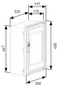
Coffret seul
