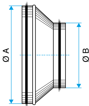
Schéma d'encombrement Réduction Conique Concentrique à joints
